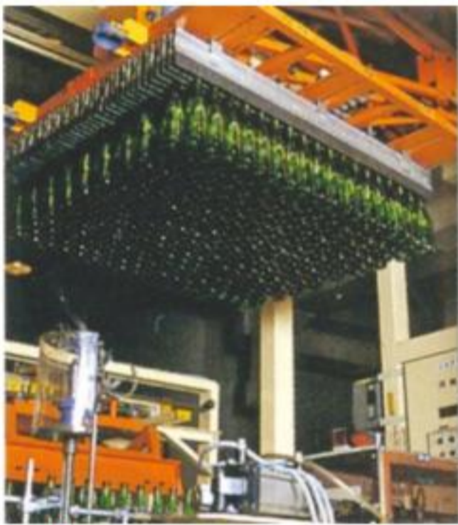
梱包するバルク包装設備。
