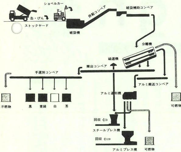
■缶・びんの選別システムのフローシート
